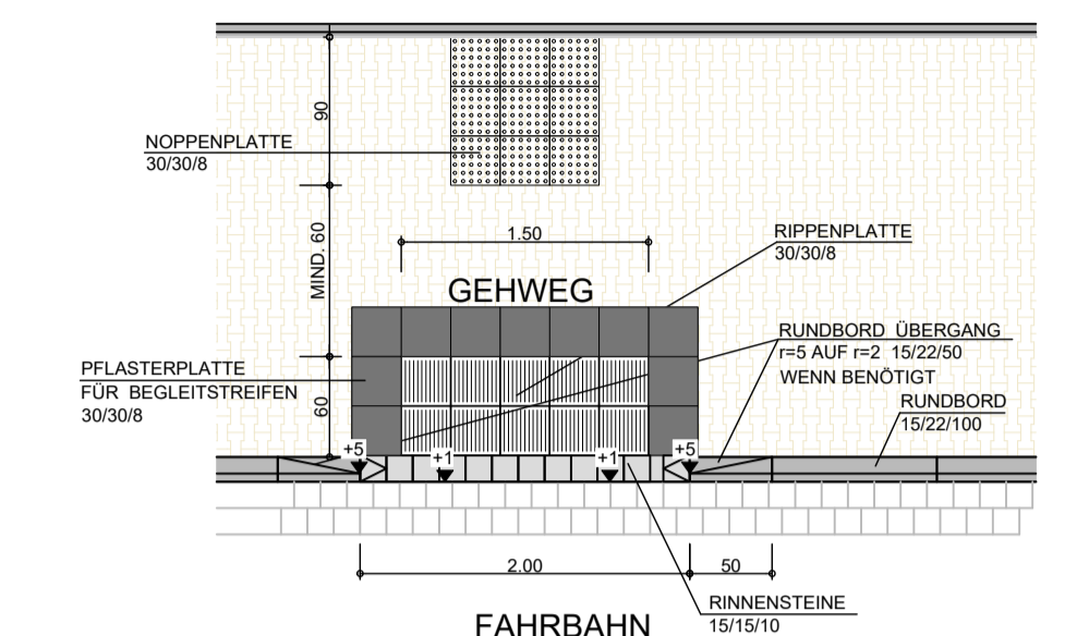
SCHEMA HÖHEN ÜBERGANG (ZUSAMMEN) M = 1:50
